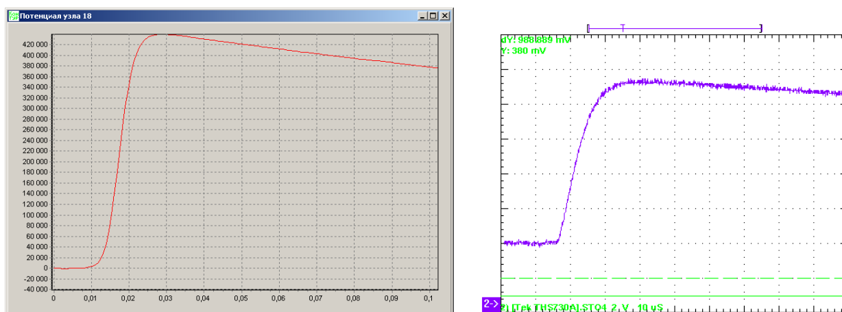
Рис. 8. Результаты определения импульсного потенциала для мачты не связанной с общим ЗУ, имеющей только собственный обособленный заземлитель: а) результат численного моделирования в ПО «Контур», б) результат имитационного моделирования с помощью ЛУГ-1М
