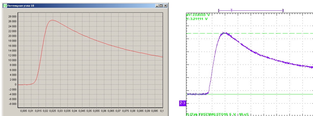
Рис. 7. Результаты определения импульсного потенциала для мачты связанной с общим ЗУ только проводником кабеля прожектора: а) результат численного моделирования в ПО «Контур», б) результат имитационного моделирования с помощью ЛУГ-1М
