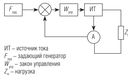
Рис. 3. Блок-схема генератора импульсов
