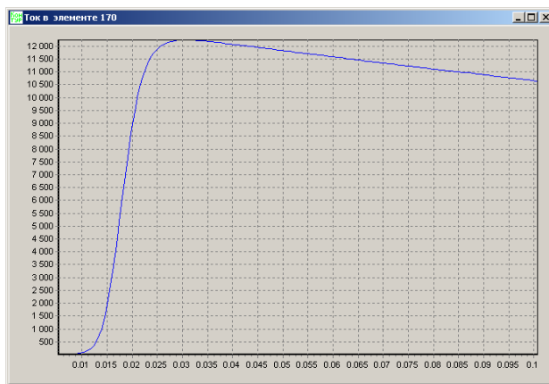
Рис. 4. Форма импульса тока 10/350 мкс, полученная при испытаниях генератора на различных объектах: вверху – осциллограммы, внизу – «эталонный» импульс 10/350 мкс
