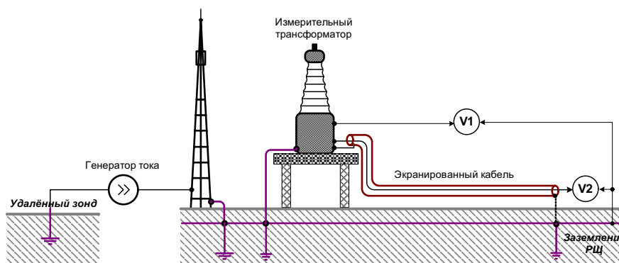
Рис. 5. Схема измерения импульсной разности потенциалов (V1) и помехи на входе аппаратуры (V2)
