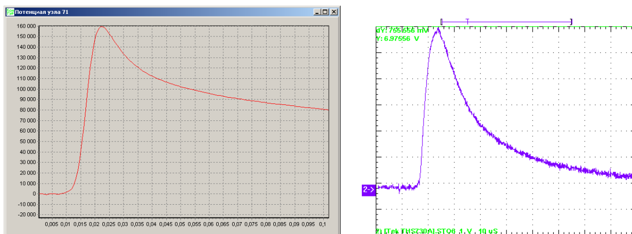
Рис. 6. Результаты определения импульсного потенциала для мачты связанной с общим ЗУ как искусственными заземлителями, так и проводником кабеля прожектора: а) результат численного моделирования в ПО «Контур», б) результат имитационного моделирования с помощью ЛУГ-1М
